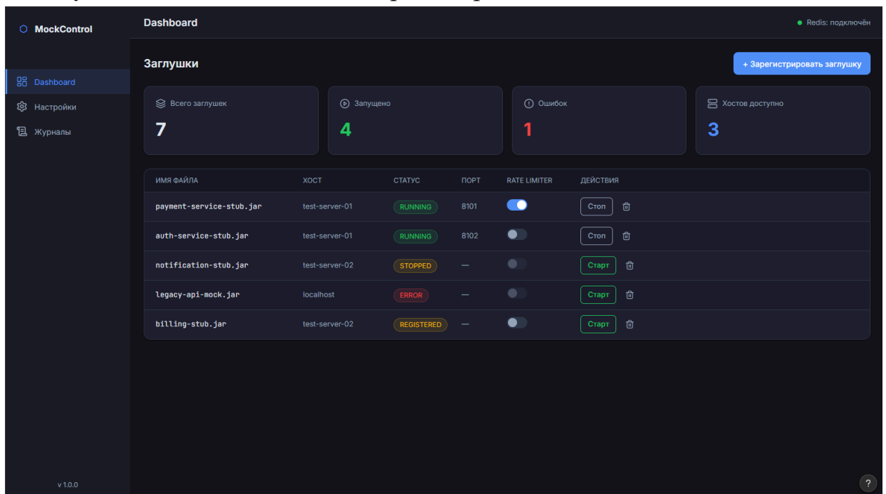
Рисунок Б.2 – Макет главной панели управления (Dashboard)
