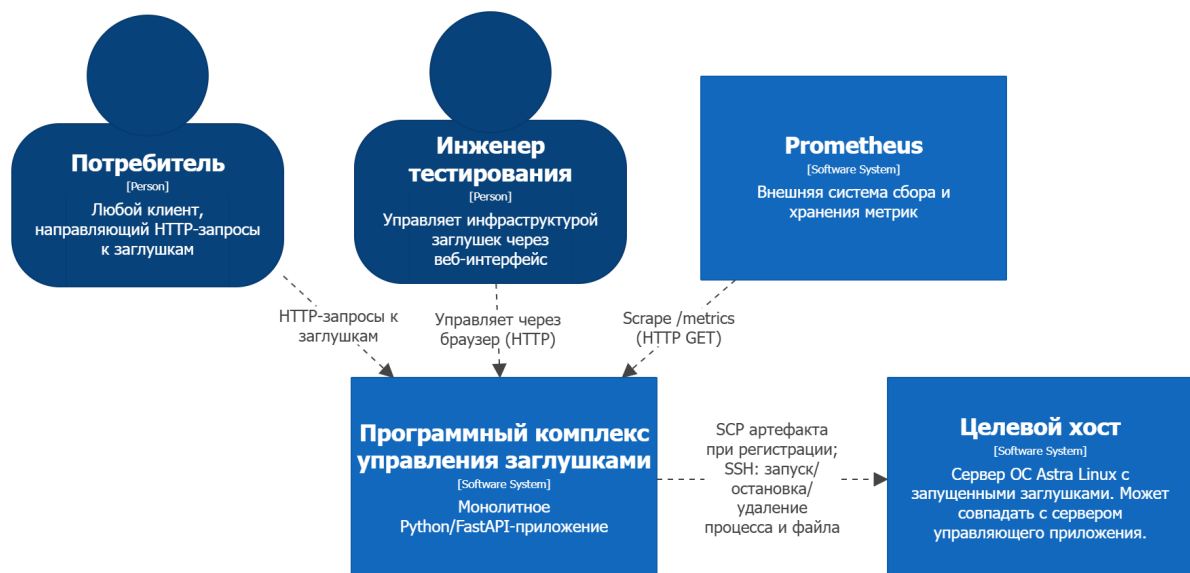
Рисунок 1 – Контекстная диаграмма системы (C4 Level 1)
