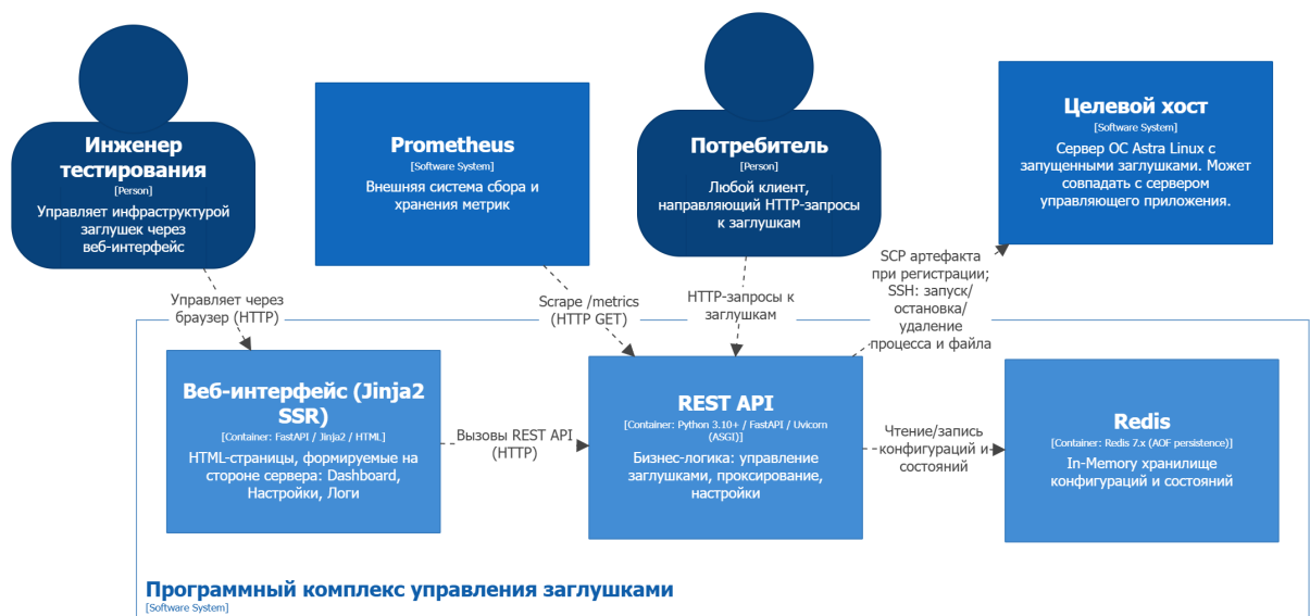
Рисунок 2 – Контейнерная диаграмма системы (C4 Level 2)
