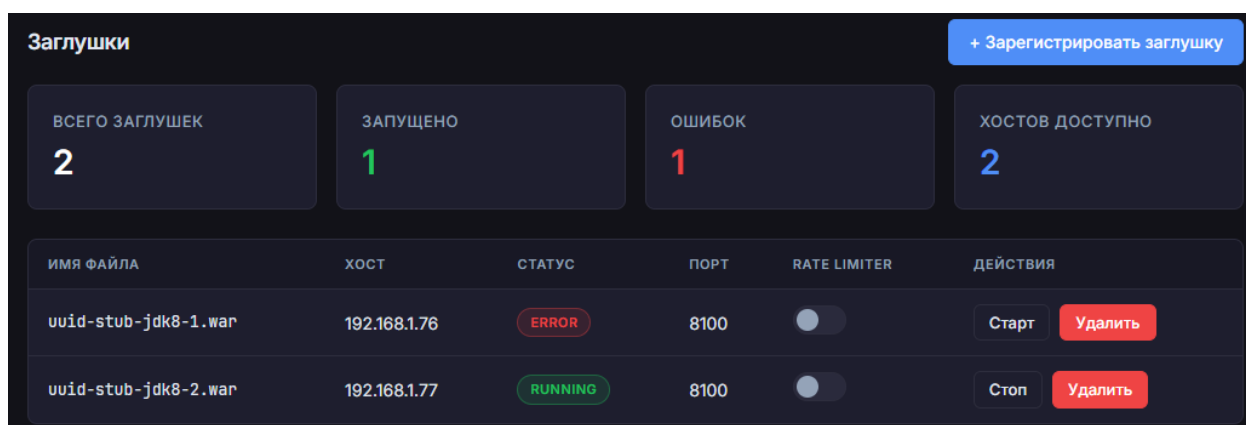
Рисунок 6 – Интерфейс панели управления: заглушка переведена в статус ERROR после обнаружения аварийного завершения процесса
