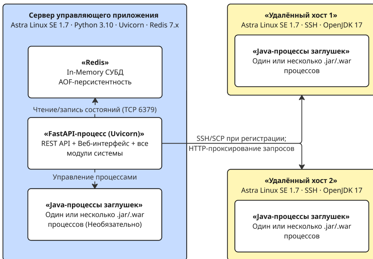
Рисунок 4 – Диаграмма развёртывания
