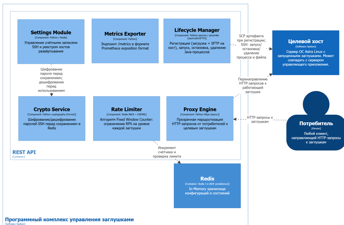
Рисунок 3 – Компонентная диаграмма REST API (C4 Level 3)
