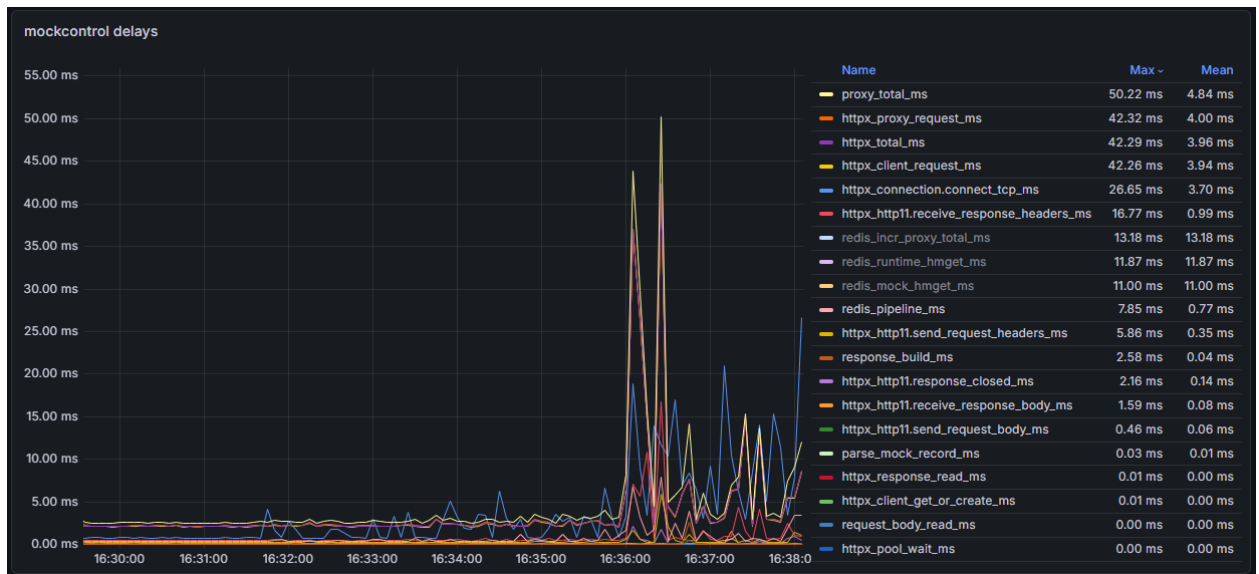
Рисунок 9 – Временные ряды метрик прокси-модуля в ходе нагрузочного испытания: нарастающая нагрузка 125–1000 RPS
