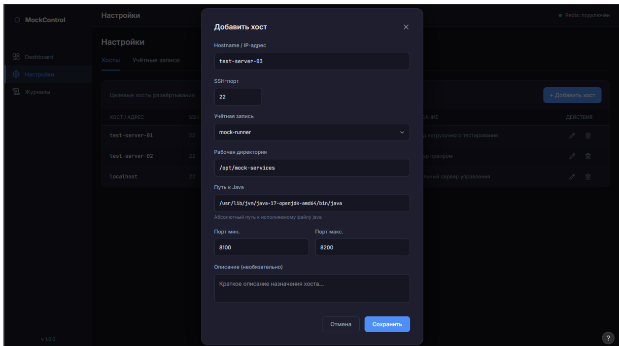
Рисунок Б.5 – Макет модального окна добавления нового хоста
